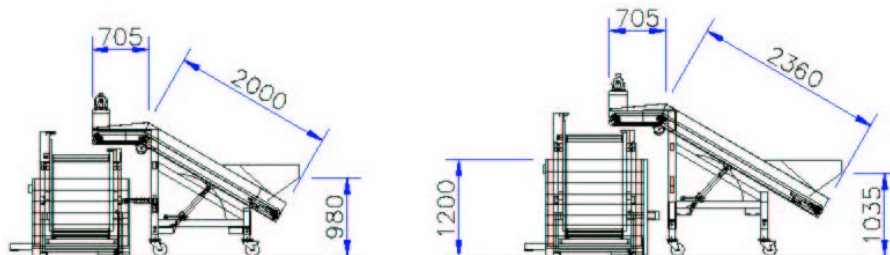
Kisten Füller mit Zuführ- Elevator
